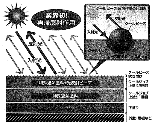
ロードクーラーの再帰反射作用
